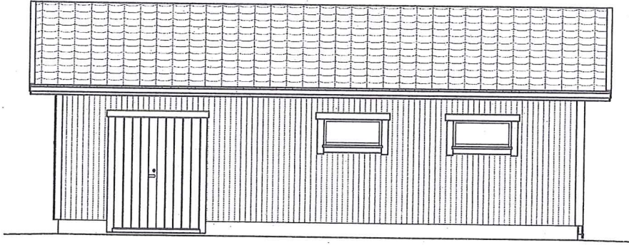
FASADERNA I FÖRHÅLLANDE TILL VÄDERSTRECK ENLIGT SITUATIONSPLANEN / ILMANSUUNNAT ASEMAPIIRROKSEN MUKAAN
